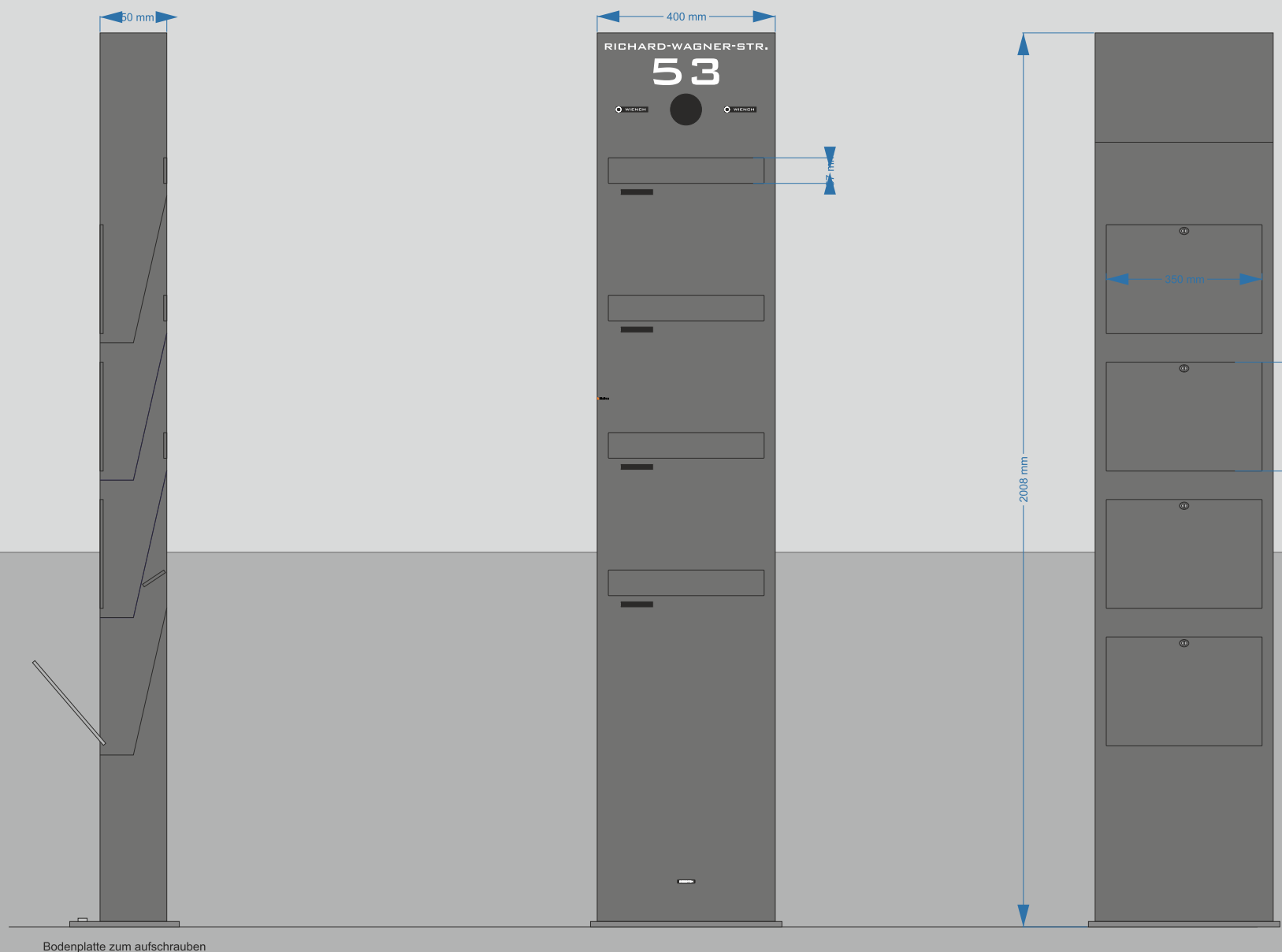
Standbriefkasten für 4 Parteien mit hinterleuchteter Straße und Hausnummer. Rückseitige Postentnahme.
